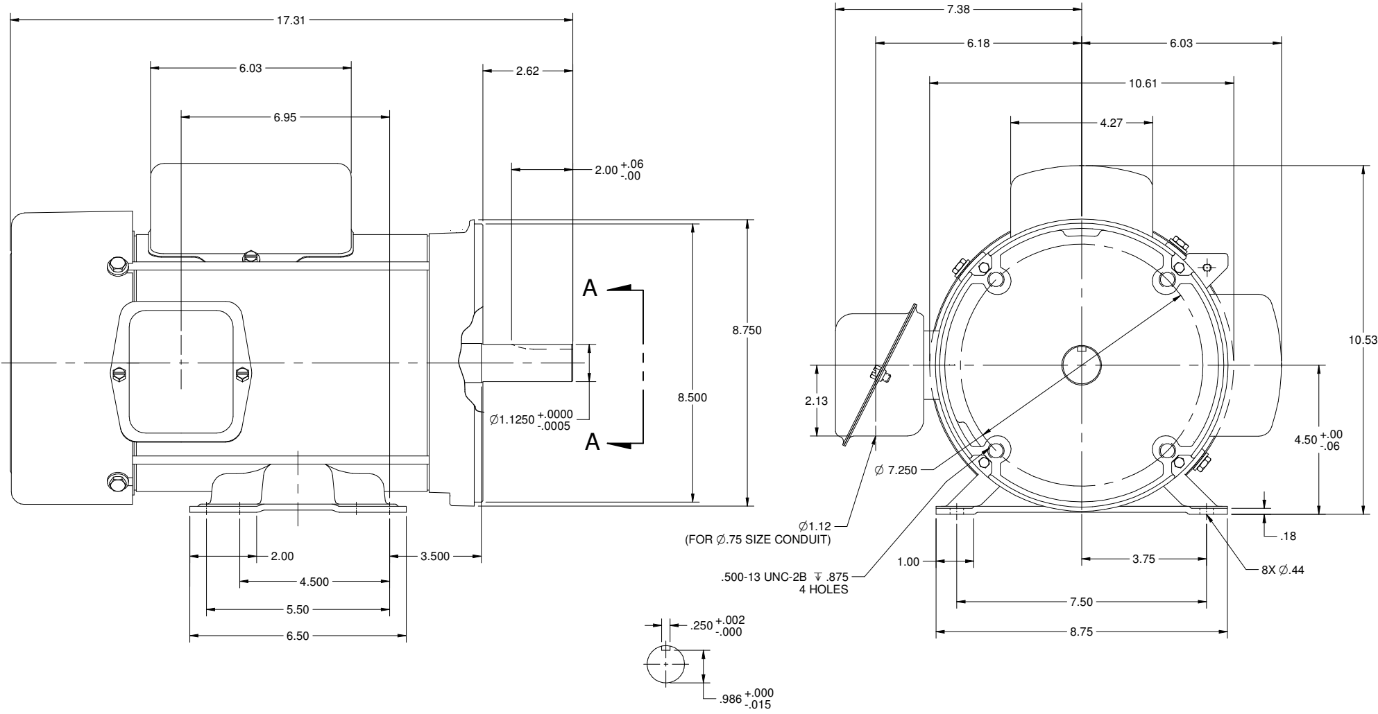
VIEW A-A
